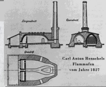
Casseler Ziegelflammofen
