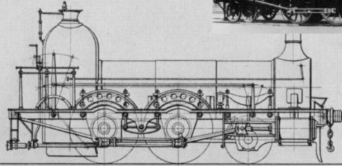
1849/50 Gemischtzug-Lokomotive Fabr.-Nr. 5 — 13
